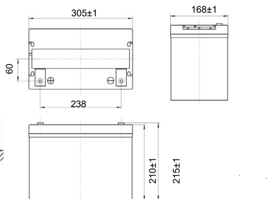
Клеммы Болт М8
